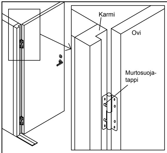
Kuva 5 Murtosuojatappien asennus
