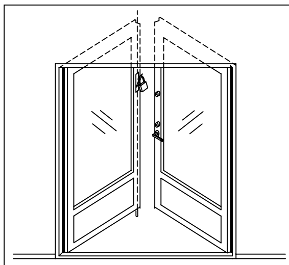
Kuva 11 Profiiliovi
