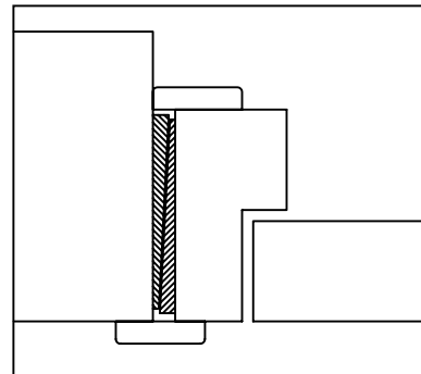
Kuva 4 Karmin kiilaus
