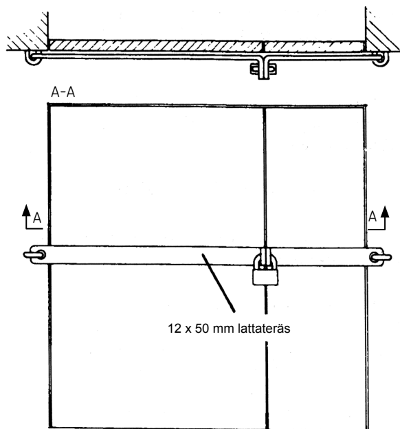
Kuva 1. Oven teräspuomi
