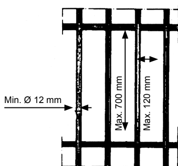
Kuva 2. Teräsristikko
