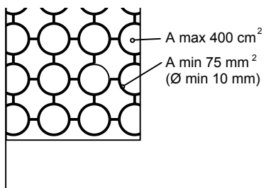
KUVA 3 MUOTOTERÄSRISTIKKO
