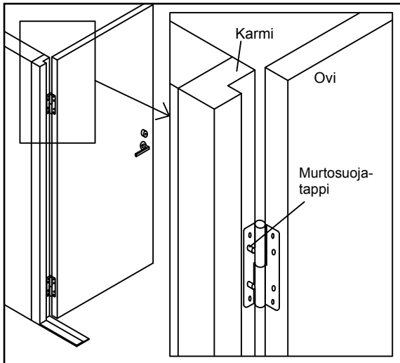
KUVA 5 MURTOSUOJATAPPIEN ASENNUS
