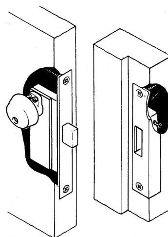
Kuva 8 Varmuuslukko vastalevyineen
