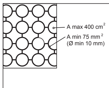
Kuva 18 Muototeräsverkko
