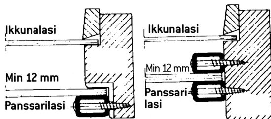
Kuva 25 Panssarilasin asennus
