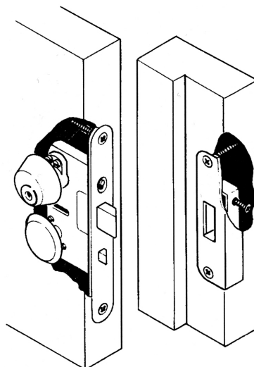
Kuva 7 Käyttölukko vastalevyineen
