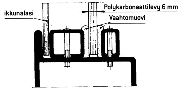
Kuva 26 Polykarbonaattilevyn joustava asennus
