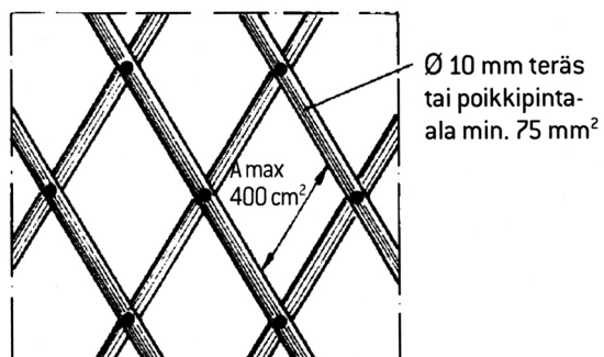
Kuva 17 Haitaristikko
