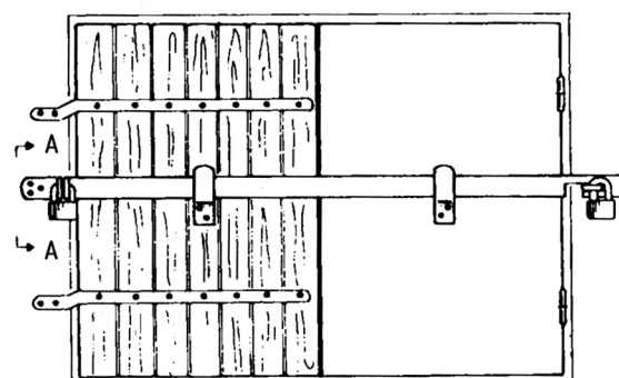
Kuva 21 Luukku
