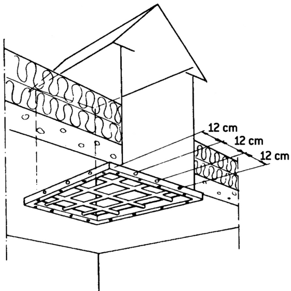
Kuva 23 Savunpoistoaukion suojaaminen teräsristikolla
