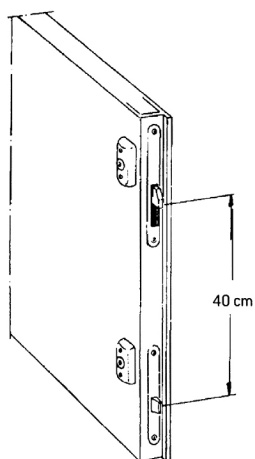
Kuva 10 Metalliprofiilioven varmuus- ja käyttölukko sekä lukkojen etäisyys toisistaan
