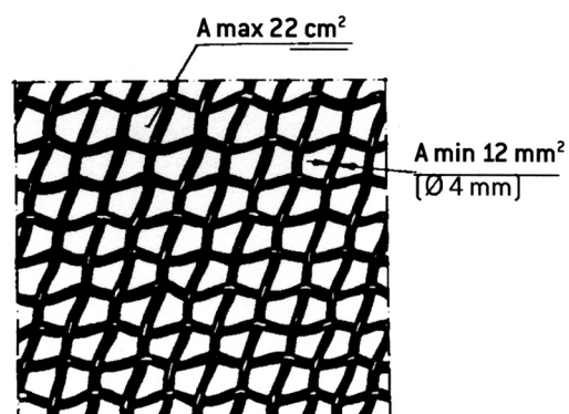
Kuva 20 Teräslankaverkko
