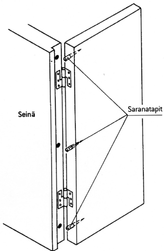
Kuva 2 A Saratappien asennus
