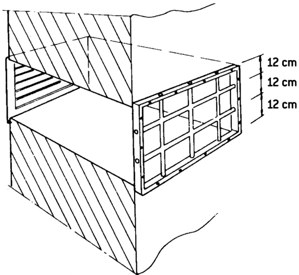
Kuva 24 Ilmanottoaukion suojaaminen teräsristikolla
