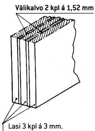
Kuva 6 Panssarilasi
