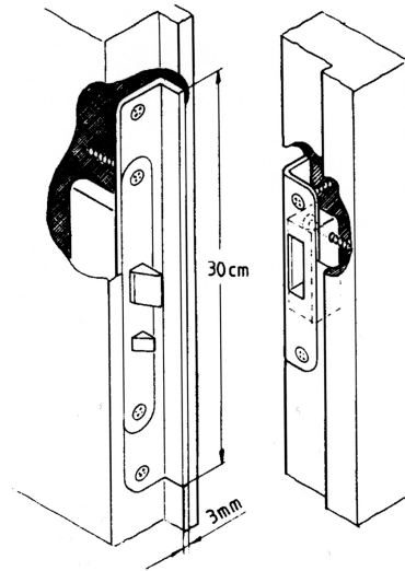
Kuva 3 A Huulletun oven rakorauta
