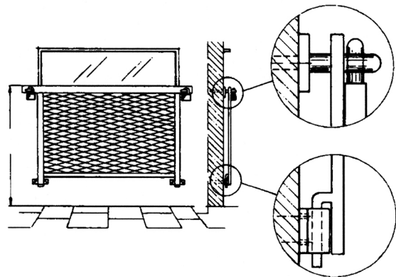
Kuva 27 Näyteikkunan suojaus ulkopuolelle asennettavalla teräsverkolla
