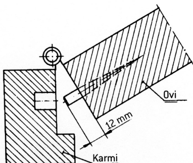
Kuva 2 B Saranatappi
