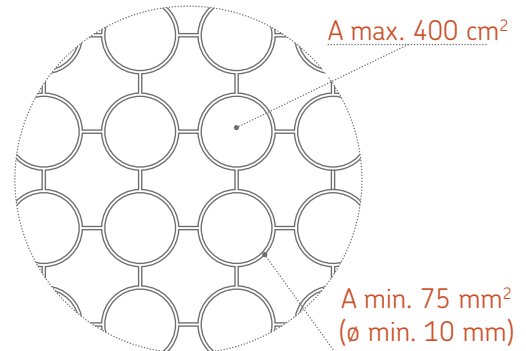
Kuva 18: Muototeräsristikko
